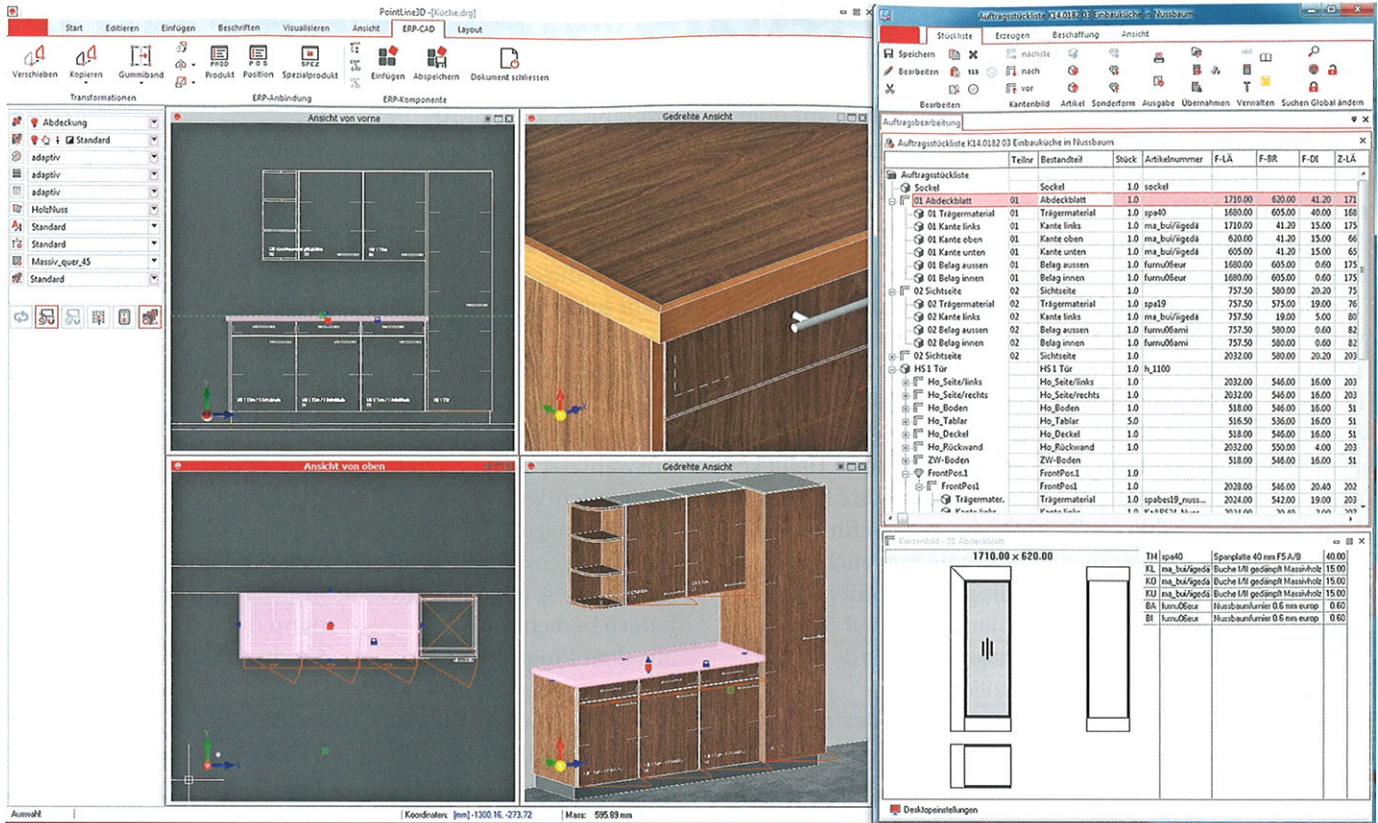
BormBusiness V1: Änderungen der Konstruktion werden in Echtzeit in der Stückliste nachgeführt
